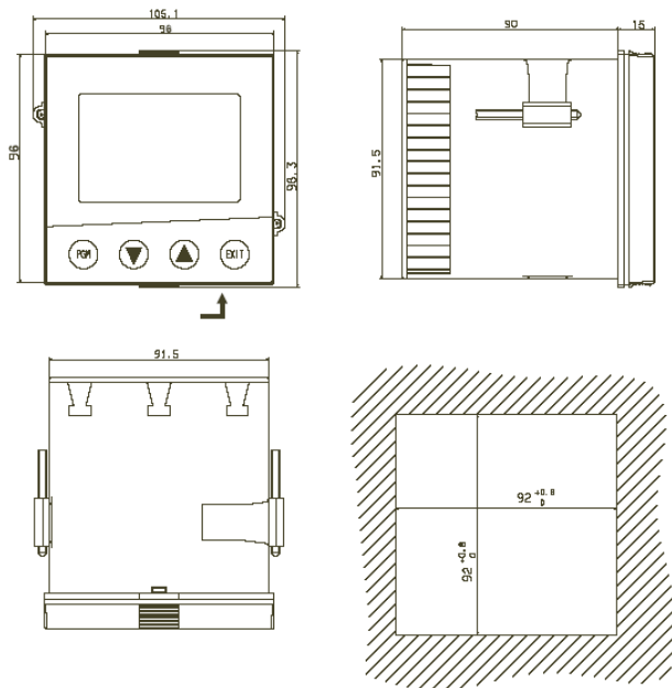
Тип 703044
