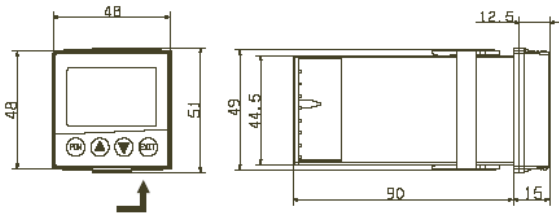
Тип 703041
