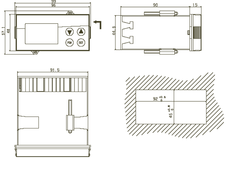
Тип 703042/43
