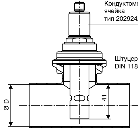
Тройник короткий аналогично DIN 11852
