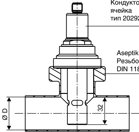
Тройник короткий аналогично DIN 11852
