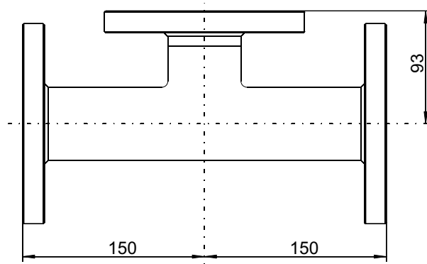
Тройник Арт.№ 20/00542773
